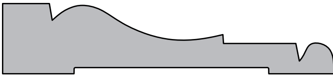
SWD 1066 | \frac{3}{4}'' \times 3\frac{1}{2}''
