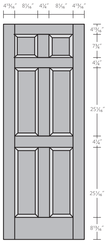
Six Panel Door
