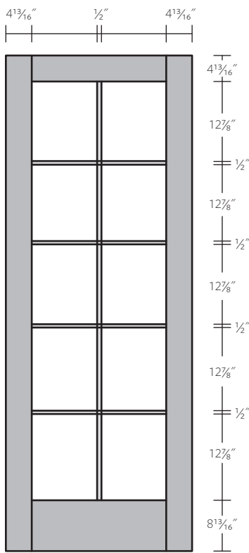
Ten Light Glass Door
