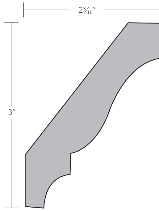
SWD 525 | \frac{3}{4}" \times 3\frac{5}{8}" | 38/52
